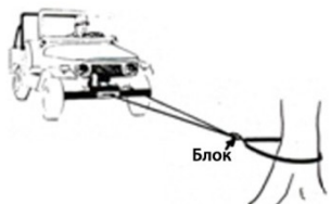
Рис. 20.6 Использование блока дает механическое усилие 2:1. К тому же вдвое уменьшается нагрузка на трос и лебедку. Соответственно, мотор будет крутить быстрее и с меньшим потреблением энергии. Можно работать с длинным тросом и не бояться перегрева мотора
