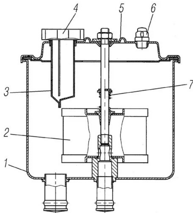
Рис. 6.14 Бачок усилителя рулевого управления: 1 – корпус; 2 – элемент фильтрующий; 3 – фильтр заливной; 4 – пробка; 5 – крышка; 6 – клапан предохранительный; 7 – пружина фильтра.
