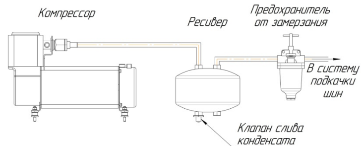
Рисунок 20.4 Схема системы предохранения СРДВШ от замерзания
