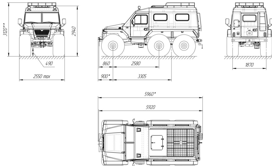
Рис. 5.3 Основные размеры ВТС ТРЭКОЛ ВЕГА
