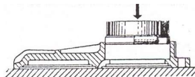
Рис.6.11 Запрессовка манжеты
