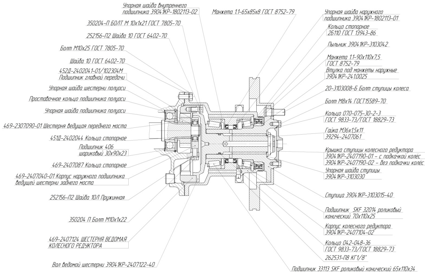
Рис. 6.12 Редуктор ТРЭКОЛ
