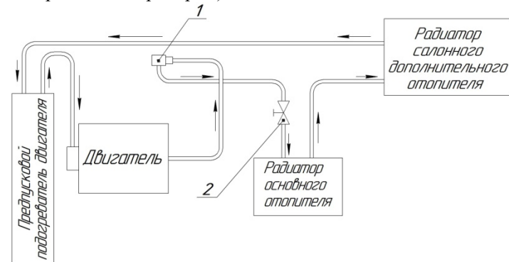
Рис. 6.20. Система отопления:
